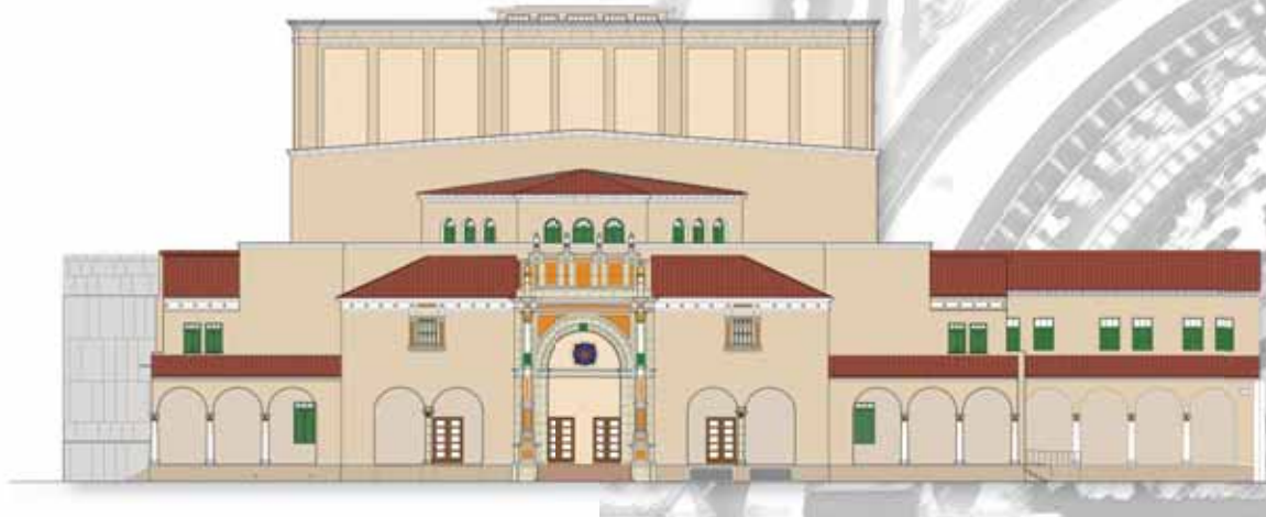
ELEVACIÓN FRONTAL
